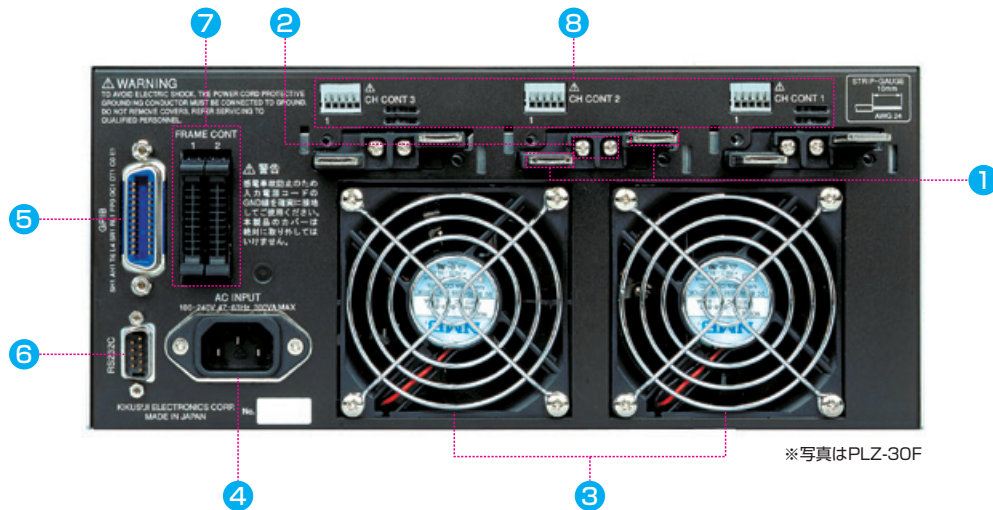
後面パネル
