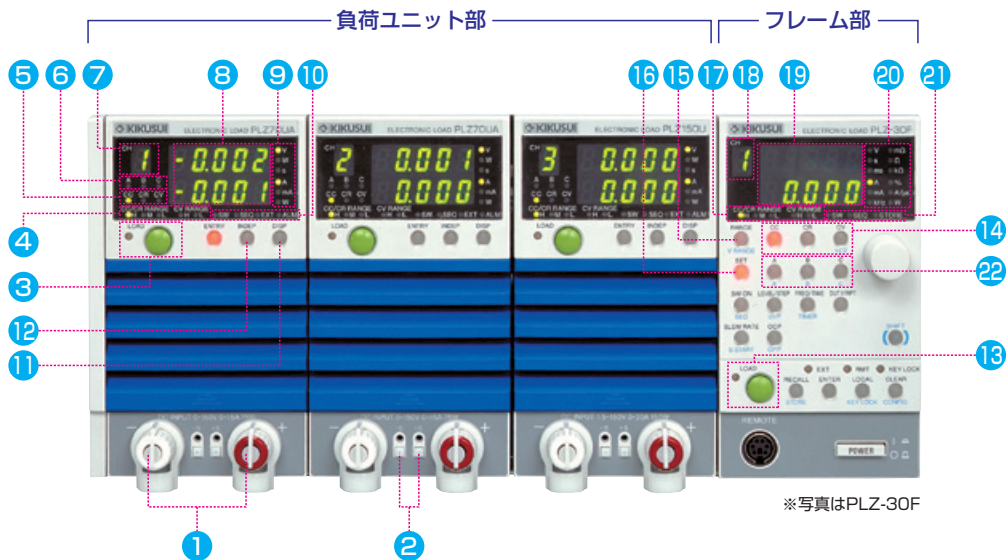
前面パネル
